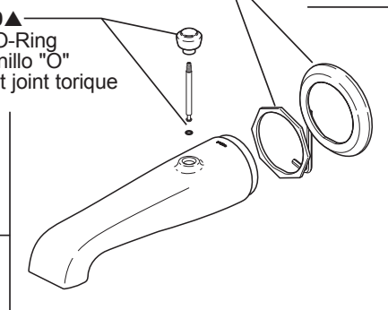
RP78581▲ Tub Spout/Pull-Up Diverter Tubo de salida para bañera/ botón desviador de alzar Bec/avec dérivation à tirette
